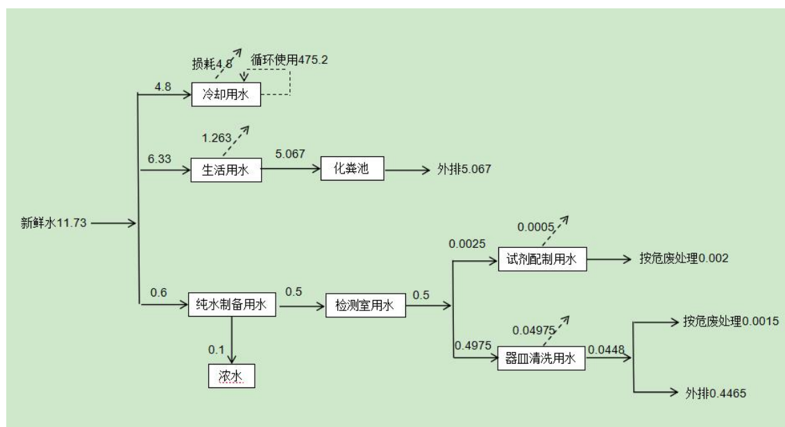
图2-1 项目水平衡图 单位m³/d
